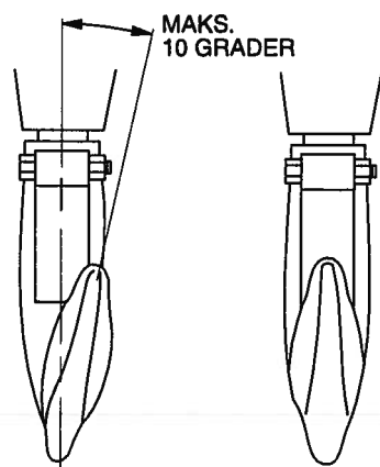
Vridd— SKAL IKKE BRUKES (Tegn. MHP0111NO)
