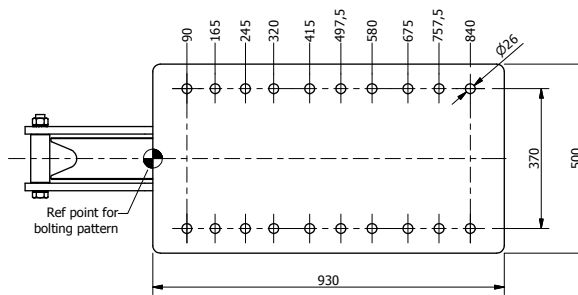
A-A ( 1 : 10 )
