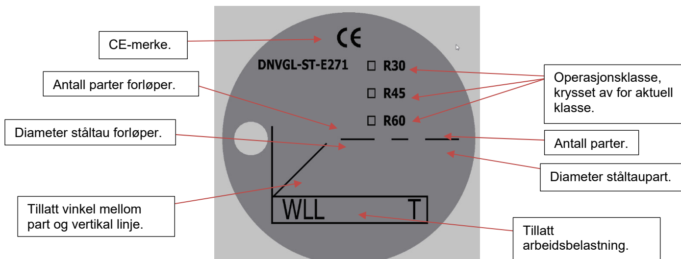
Figur 4A: Forside av merkeplate iht. DNVGL-ST-E271.
