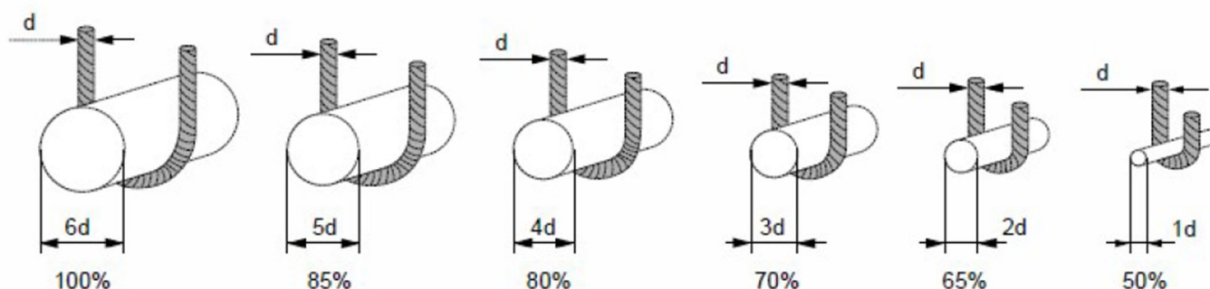
Figur 7: Bøyingsdiameterers påvirkning på WLL.
