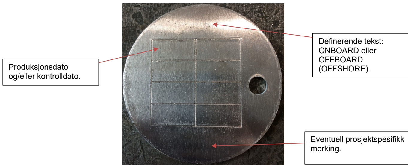
Figur 3B: Bakside av merkeplate.
