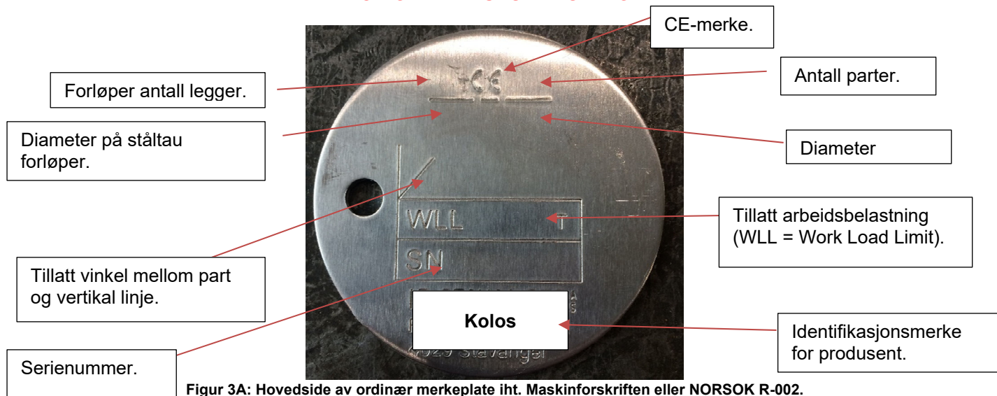
Figur 3A: Hovedside av ordinær merkeplate iht. Maskinforskriften eller NORSOK R-002.
