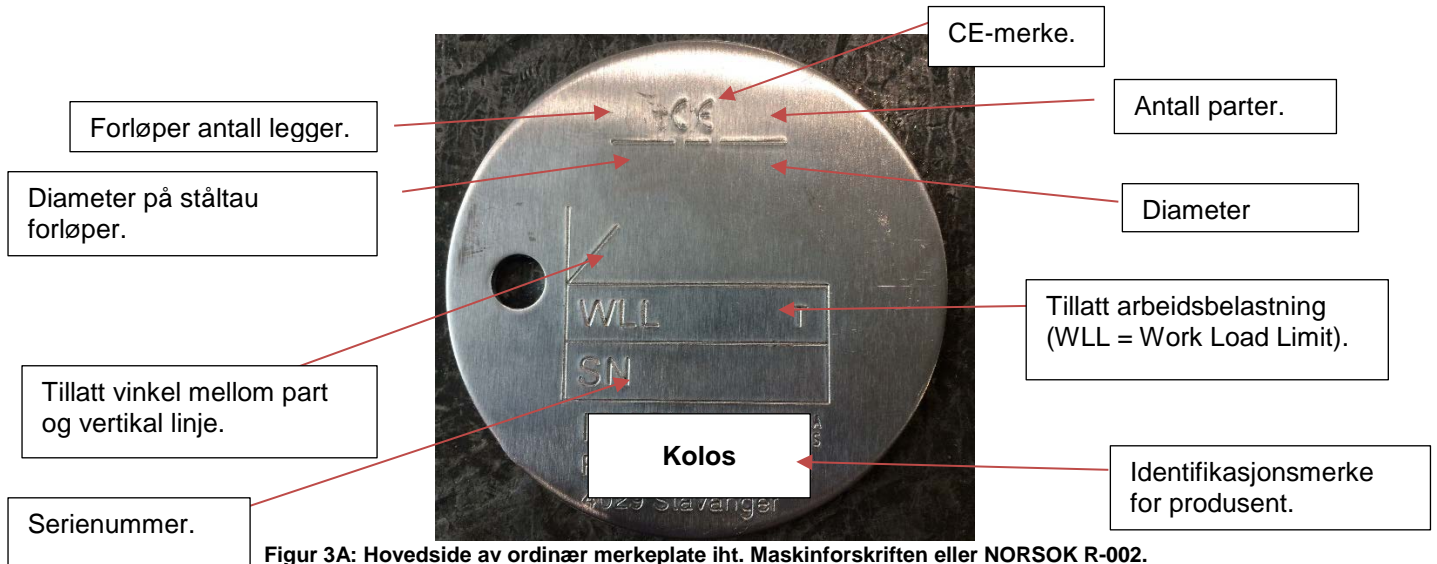
Figur 3A: Hovedside av ordinær merkeplate iht. Maskinforakriften eller NORSOK R-002.
